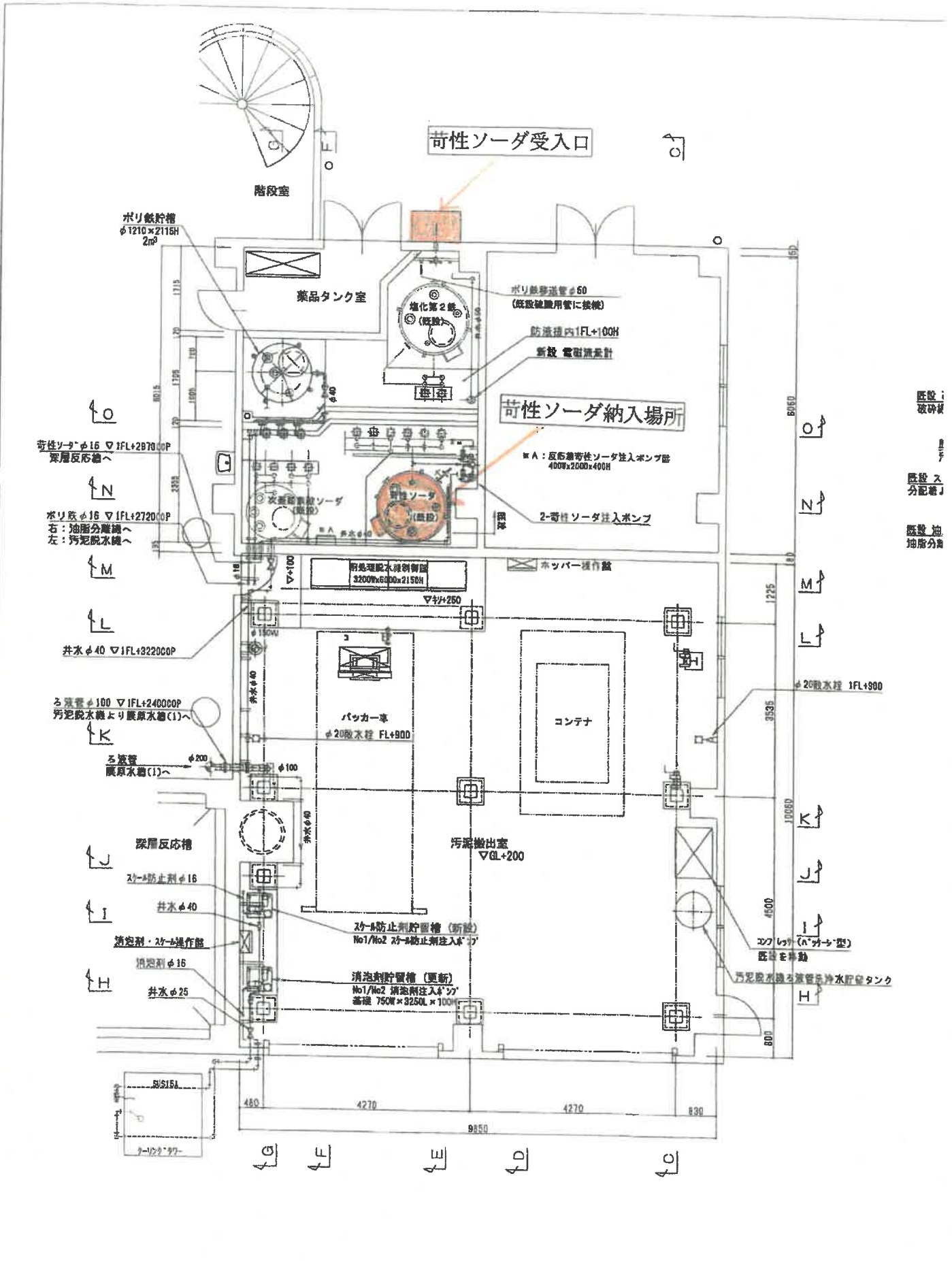
1階下部平面図 S=1/50
